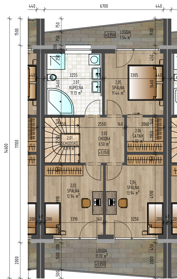
DOM S - PÔDORYS 2.NP
