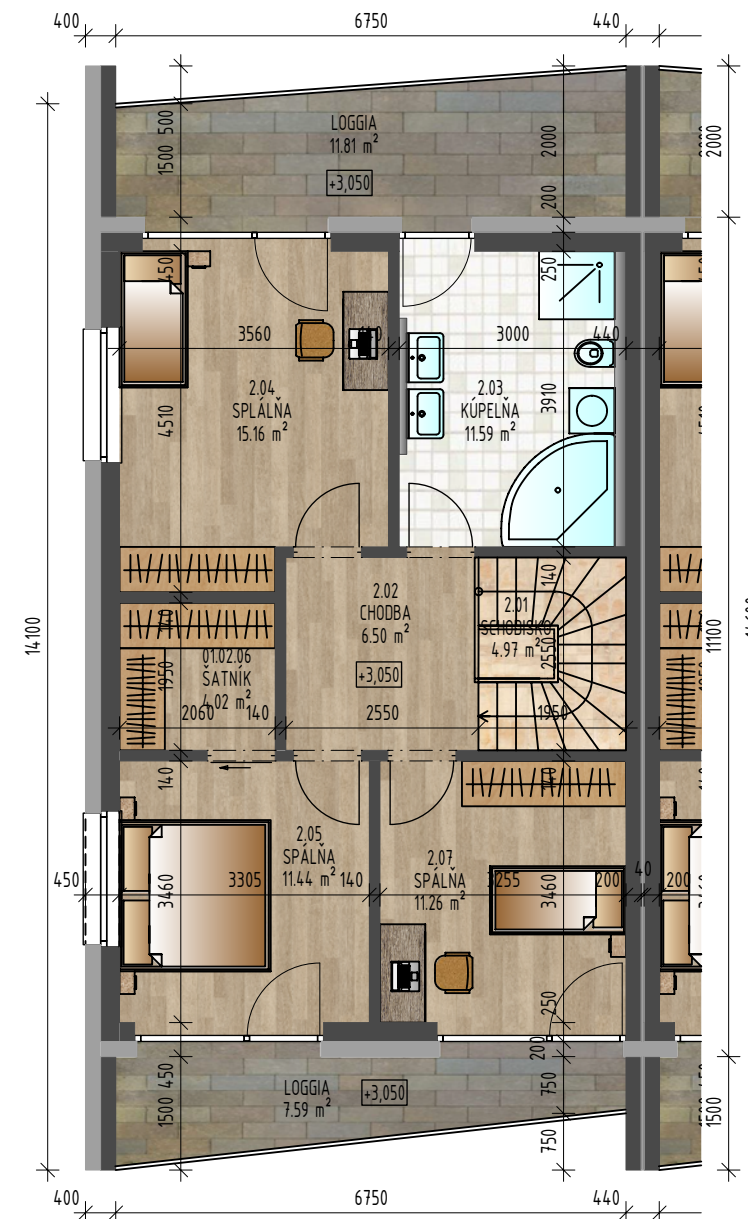
DOM A - PÔDORYS 2.NP
